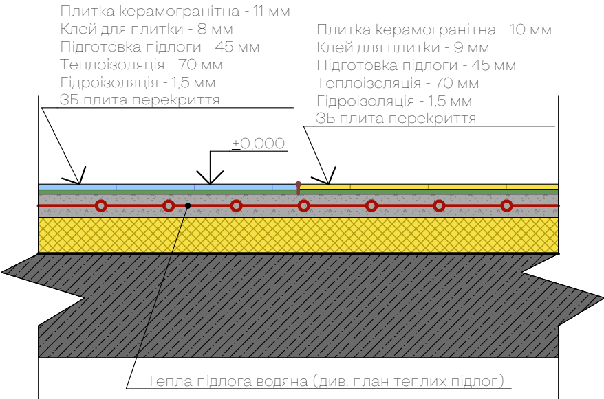
Розріз підлоги-3 Деталь 1:10
