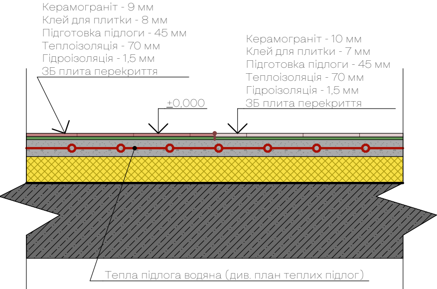
Розріз підлоги-5 Деталь 1:10
