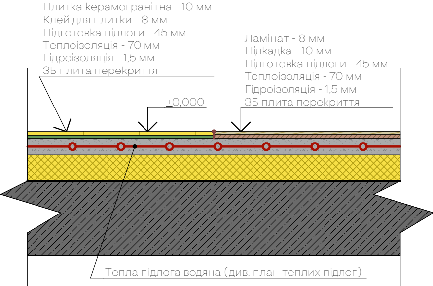
Розріз підлоги-2 Деталь 1:10
