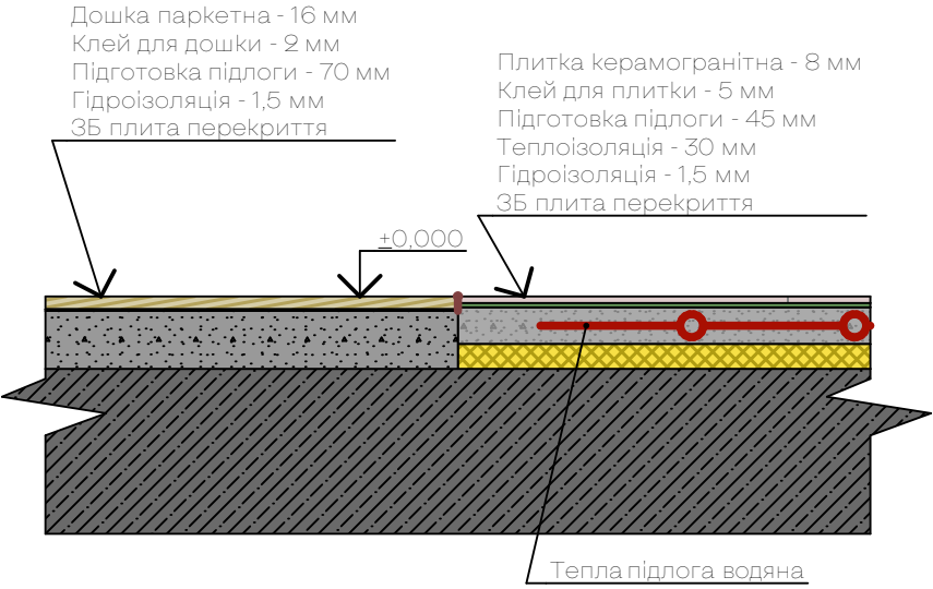
Розріз підлоги - 1 Деталь 1:10
