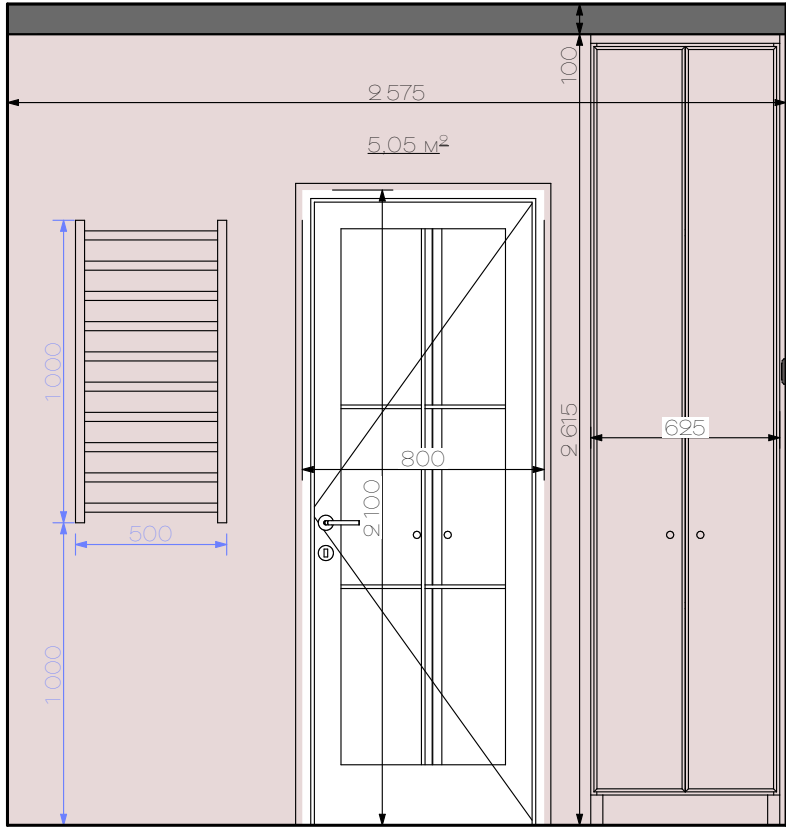
CB-1 04 CB-1 1:25
