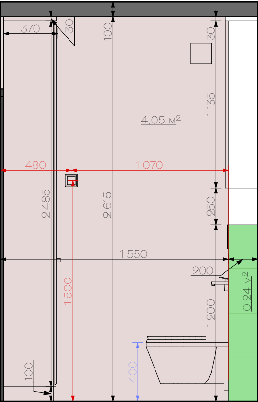
CB-1 01 CB-1 1:25
