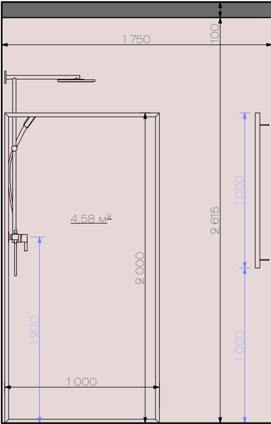
CB-1 03 CB-1 1:25
