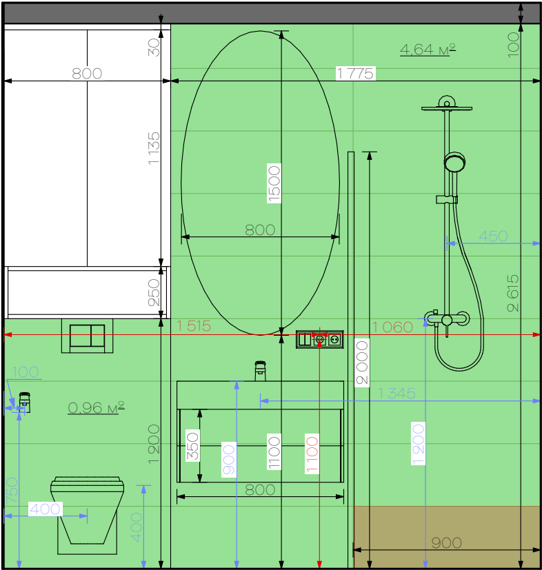
CB-1 02 CB-1 1:25
