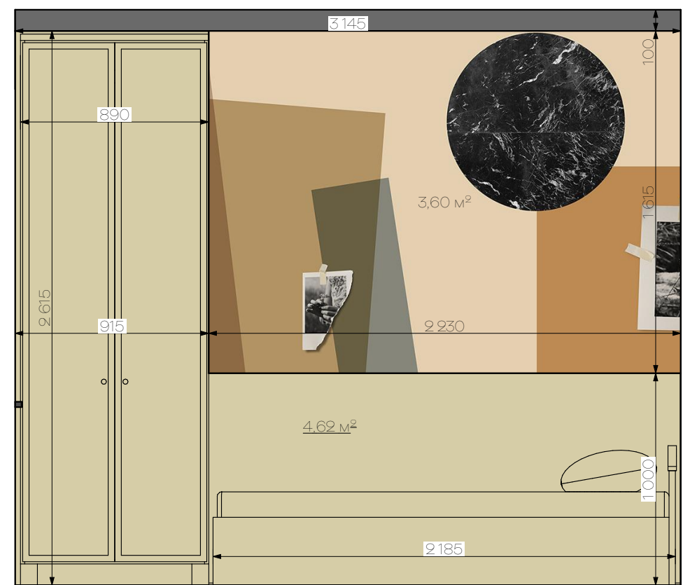
ДИТ-1.01 ДИТ 1:25
