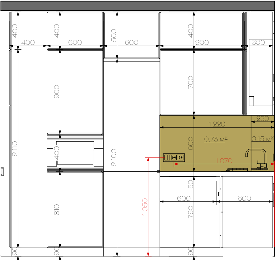
КВХ-1.02 КВХ 1:25
