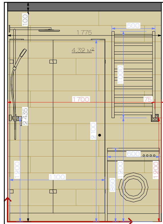
CB-1 01 CB-1 1:25
