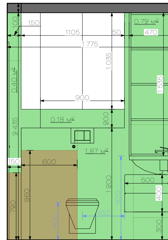
CB-1 03 CB-1 1:25
